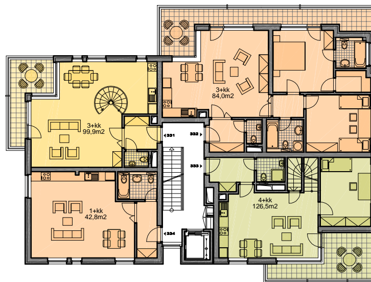
spodní úroveň / lower level
