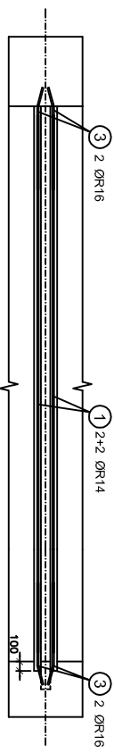
DOLNÍ VÝZTUŽ TRÁMKU
