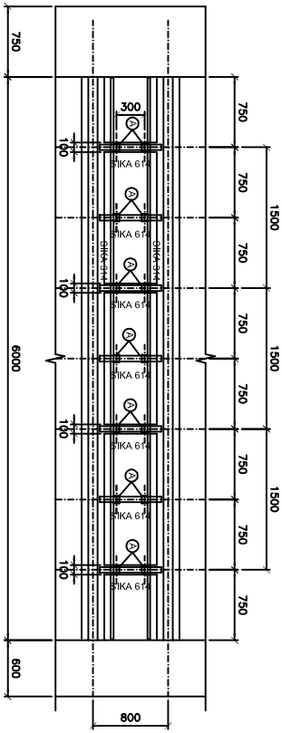
PŮDORYS - SÍKA LAMELY
