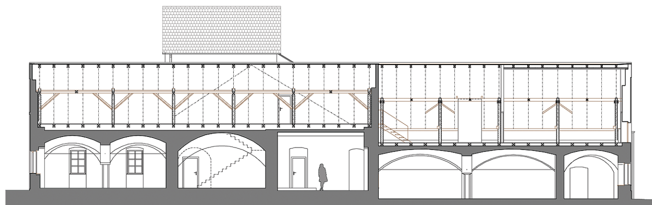
ŘEZ C-C
