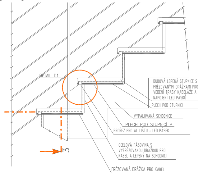
ČELNÍ POHLED
