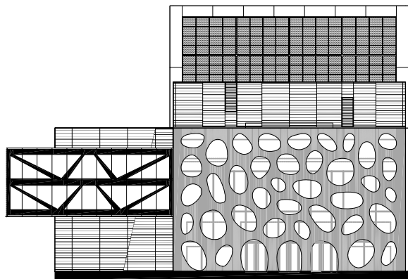
divadelní budova - pohled jižní
