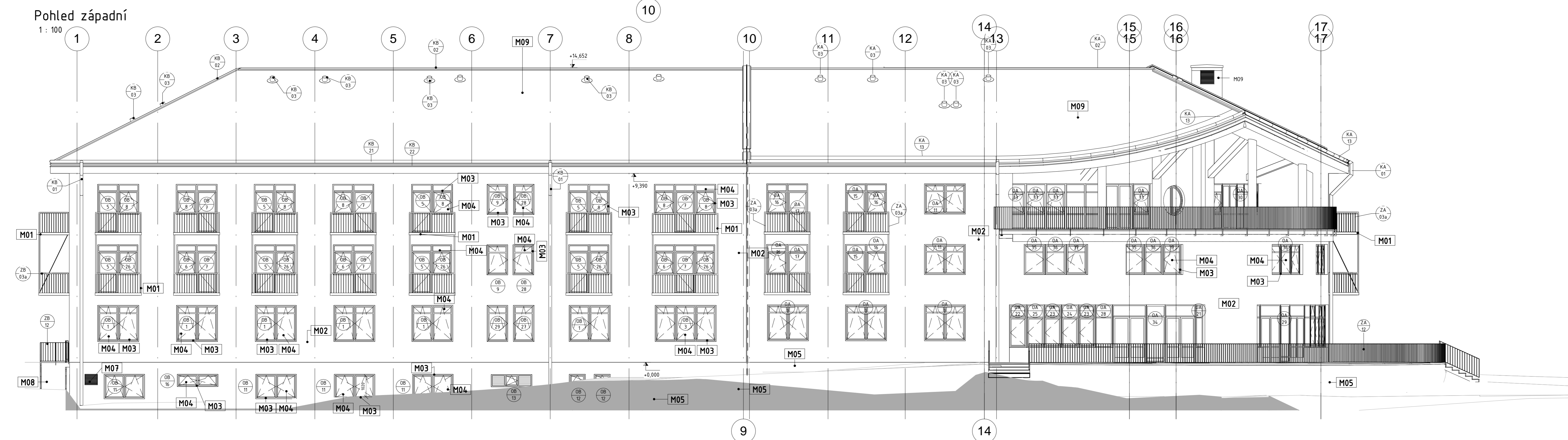
Pohled západní 1:100
