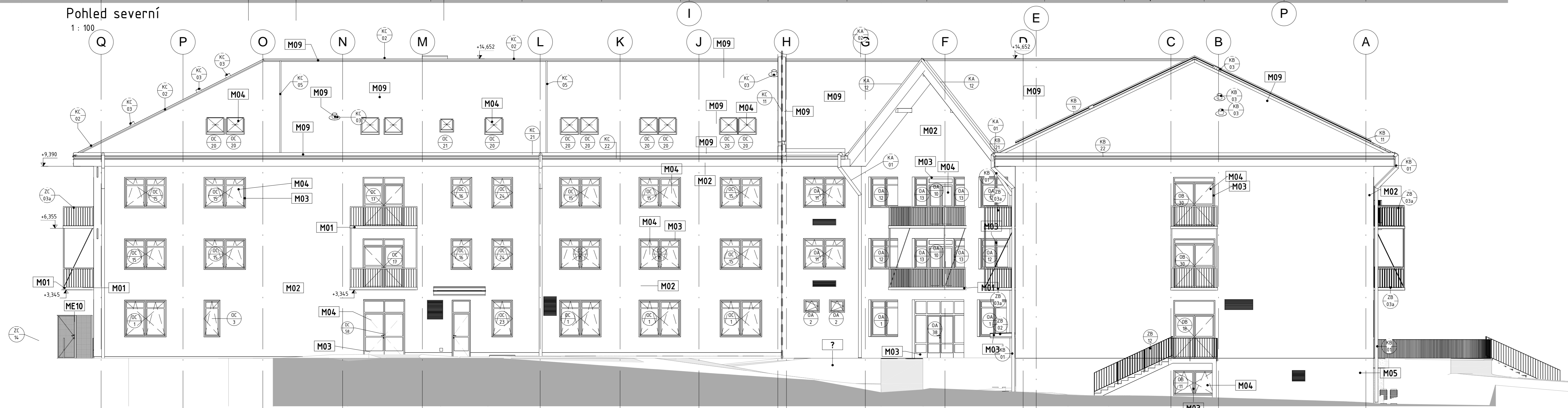
Pohled východní 1:100
