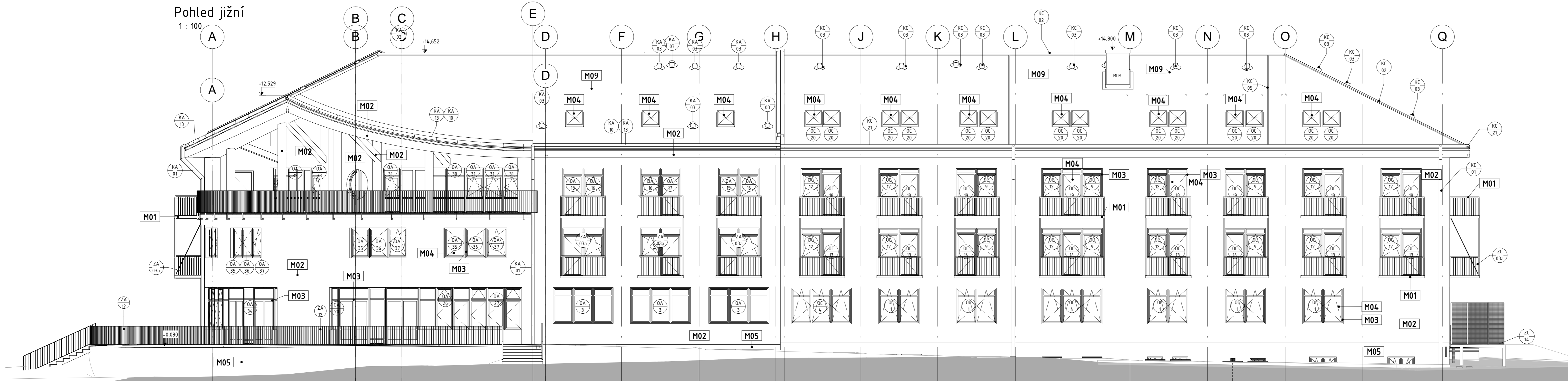
Pohled severní 1:100
