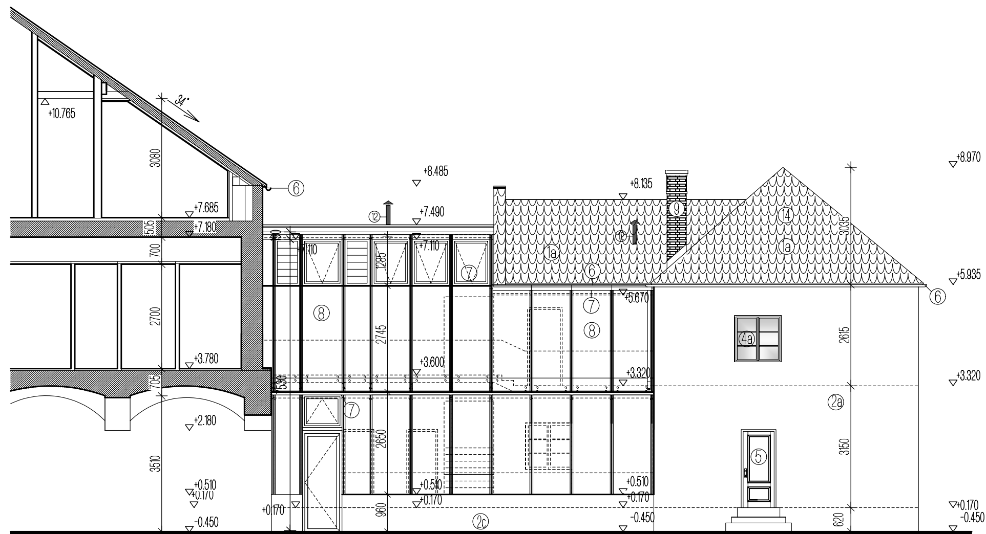
POHLED ZÁPADNÍ DÍLČÍ
