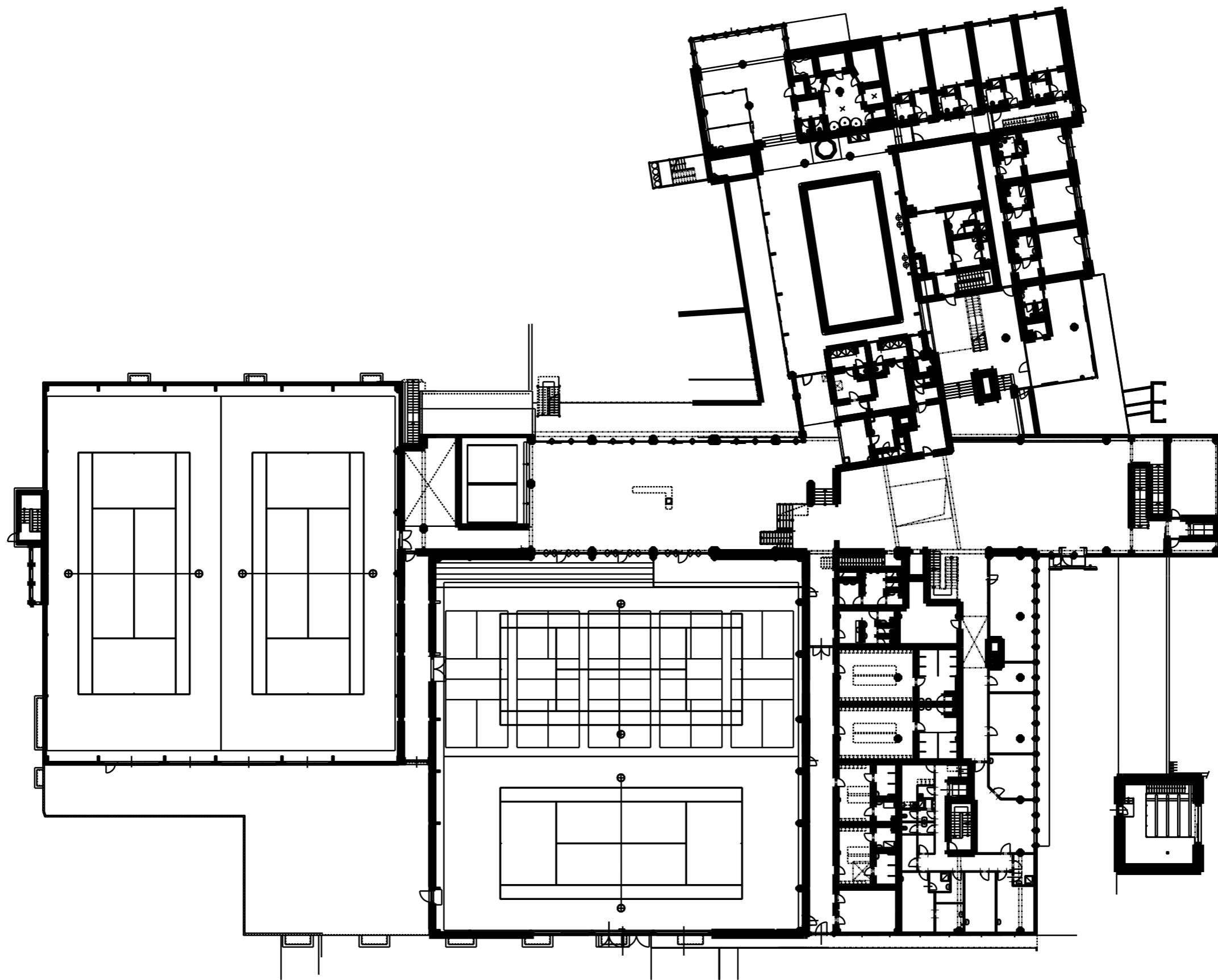
Sportovně relaxační komplex Praha - Benice 1.NP
