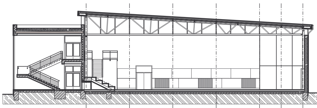
PAVILON F - ŘEZ
