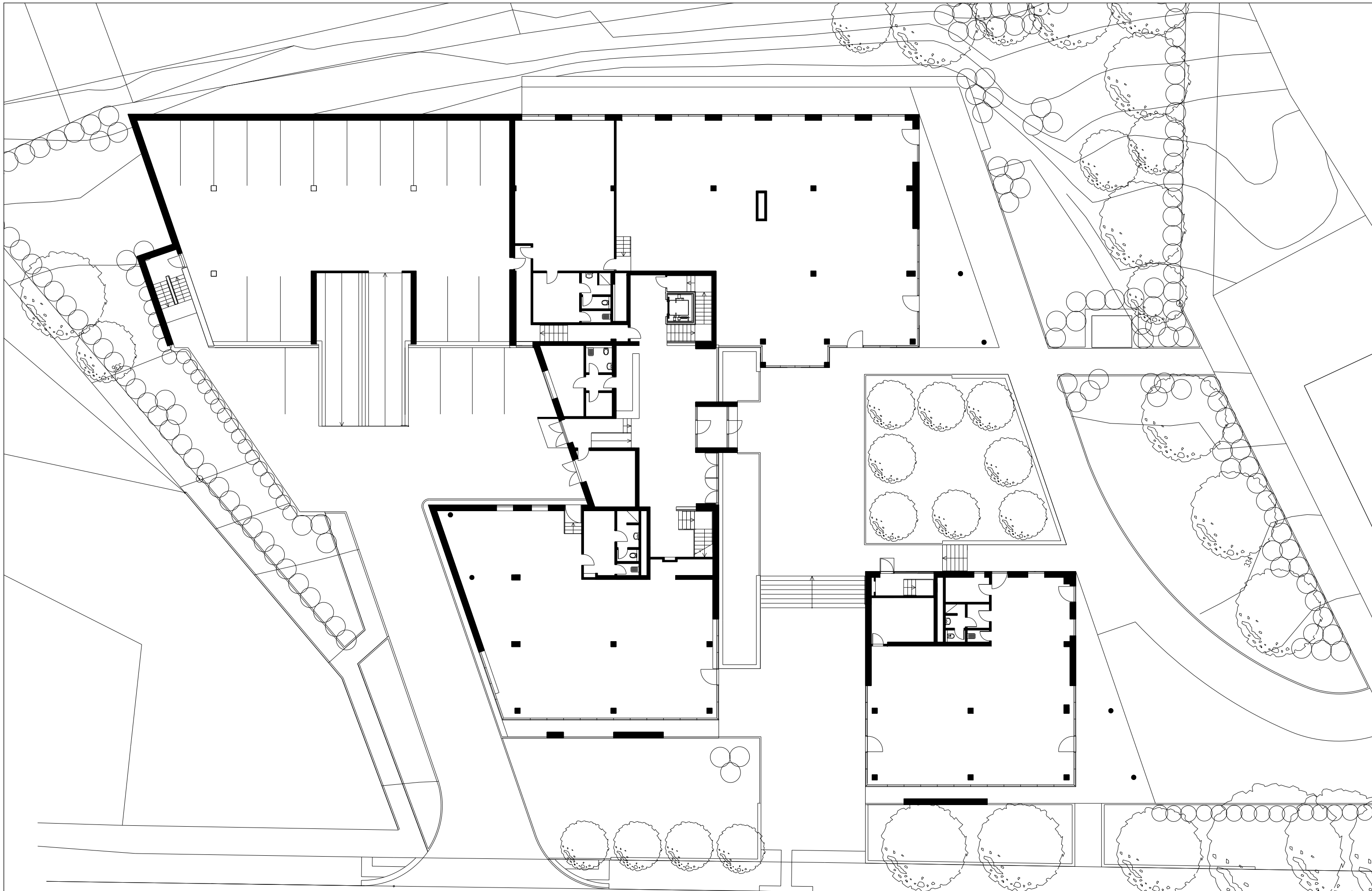
PŘÍLOHA 3 PŮDORYS 1.NADZEMNÍ PODLAŽÍ M 1:250
