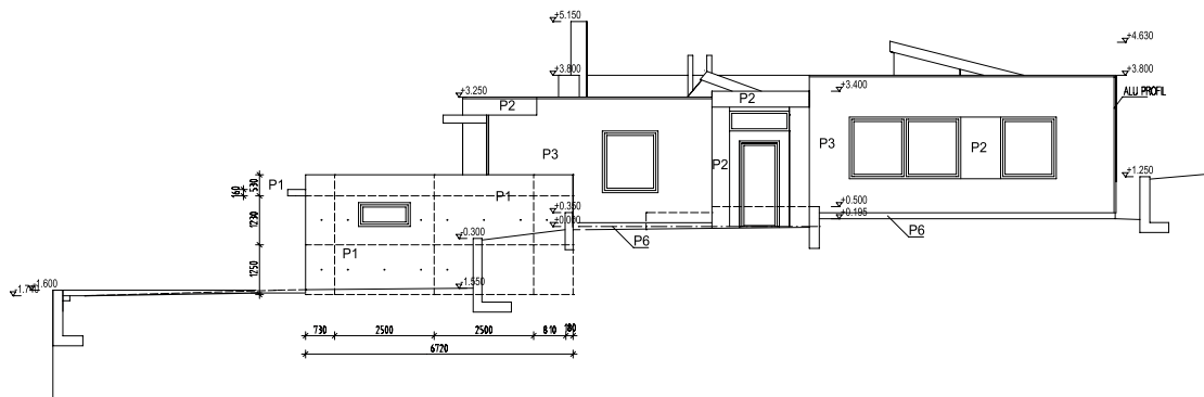
POHLED VÝCHODNÍ
