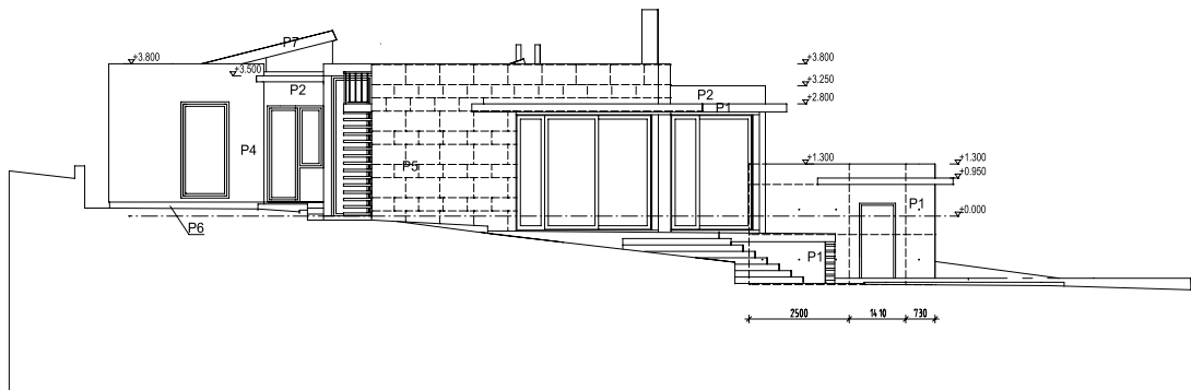
POHLED ZÁPADNÍ
