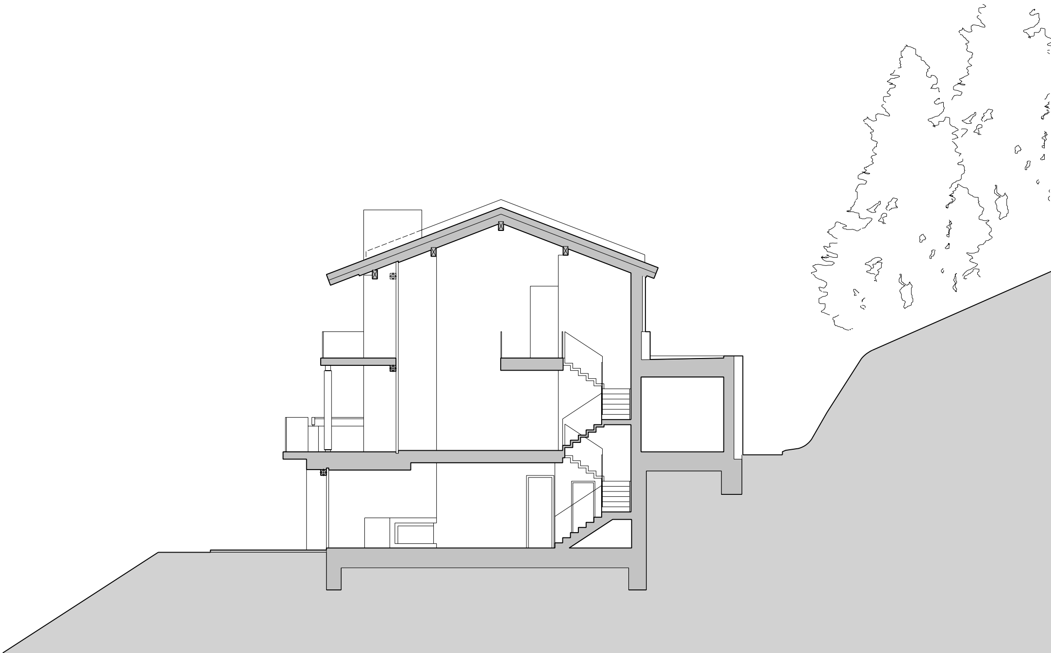
RODINNÝ DŮM KRKONOŠE PŘÍČNÝ ŘEZ M 1:125
