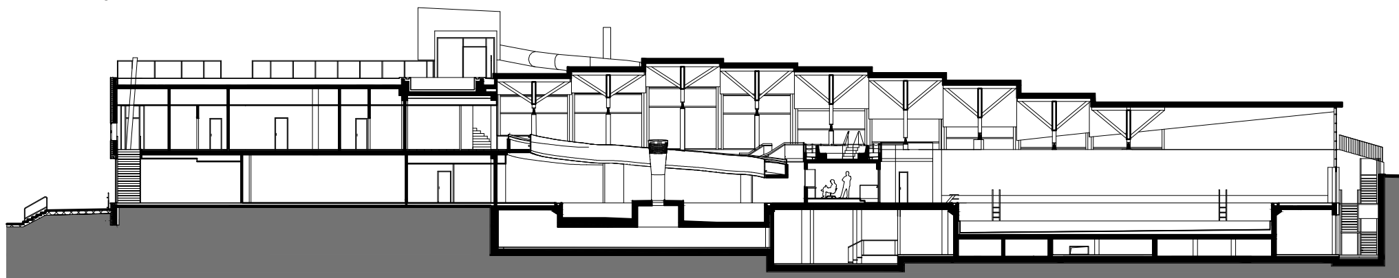
ŘEZ PODÉLNÝ
