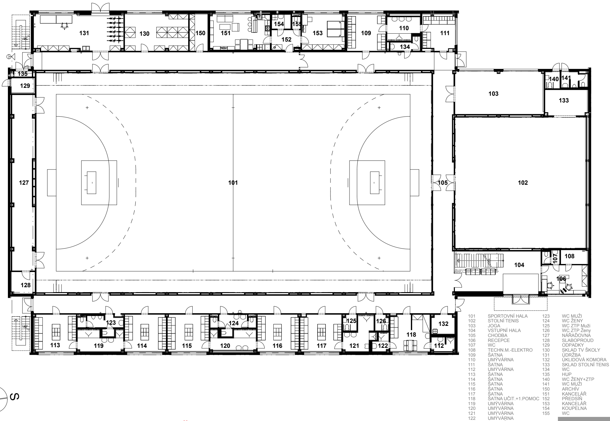
Multifunkční sportovní hala SKUTEČ - půdorys 1.NP M 1:250
