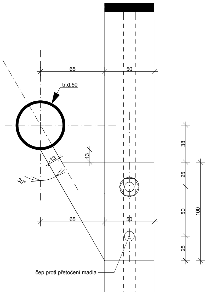
Detail podpěry madla M 1:2
