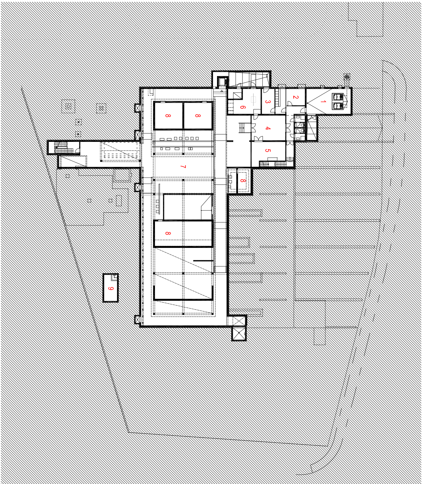
KRYTÝ PLYVECKÝ BAZÉN V LITOMÝŠLI PŮDORYS 1. PP
