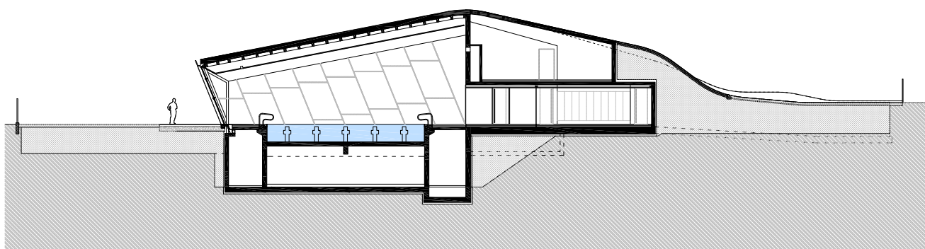
KRYTÝ PLAVECKÝ BAZÉN V LITOMÝŠLI CHARAKTERISTICKÉ ŘEZY
