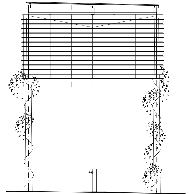
POHLED BOČNÍ
