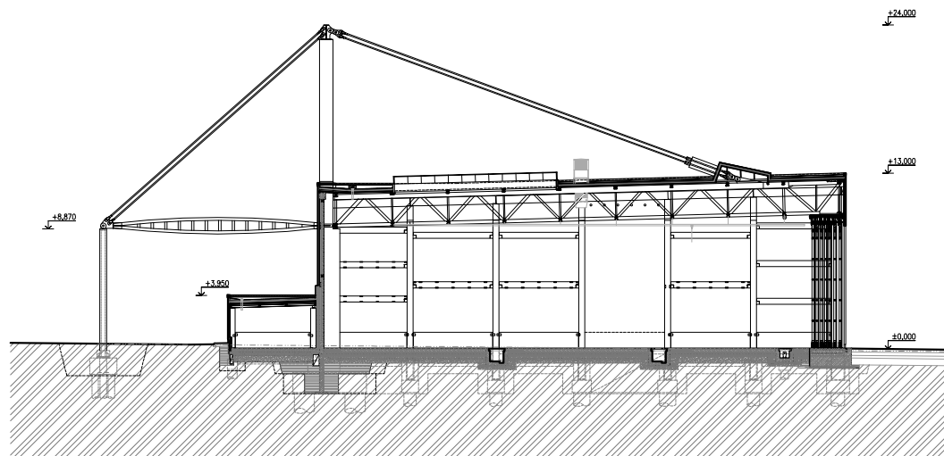
PŘÍČNÝ ŘEZ - HANGÁROVOU HALOU
