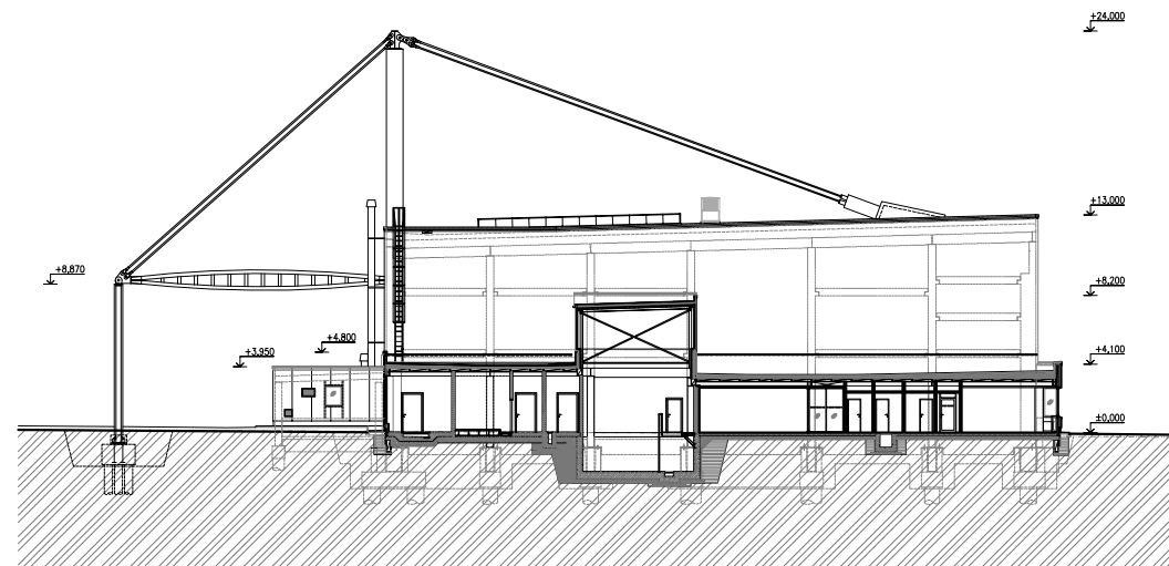
PŘÍČNÝ ŘEZ - PŘÍSTAVEK
