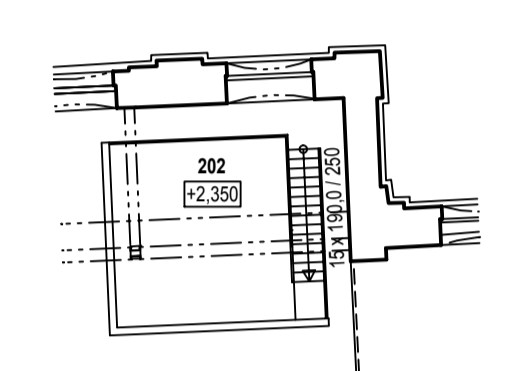
PŮDORYS GALERIE V ÚSTŘEDNĚ
