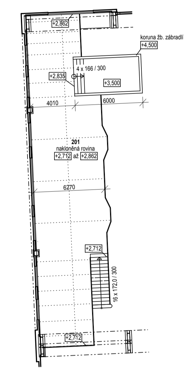
PŮDORYS GALERIE VE DVOJHALÍ
