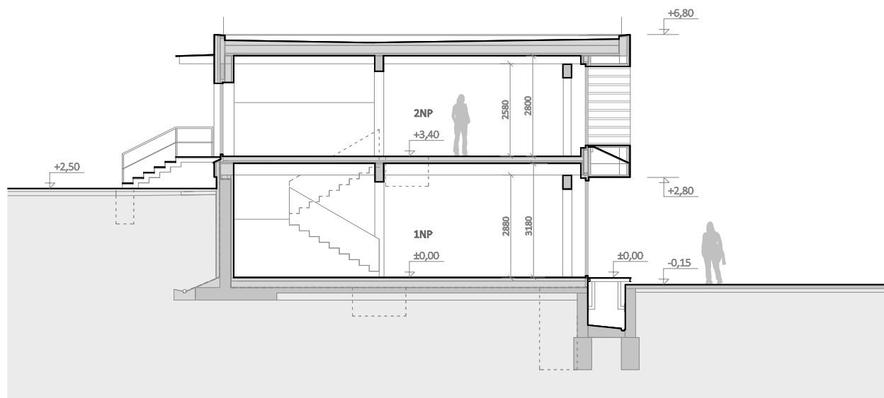
řez příčný A
