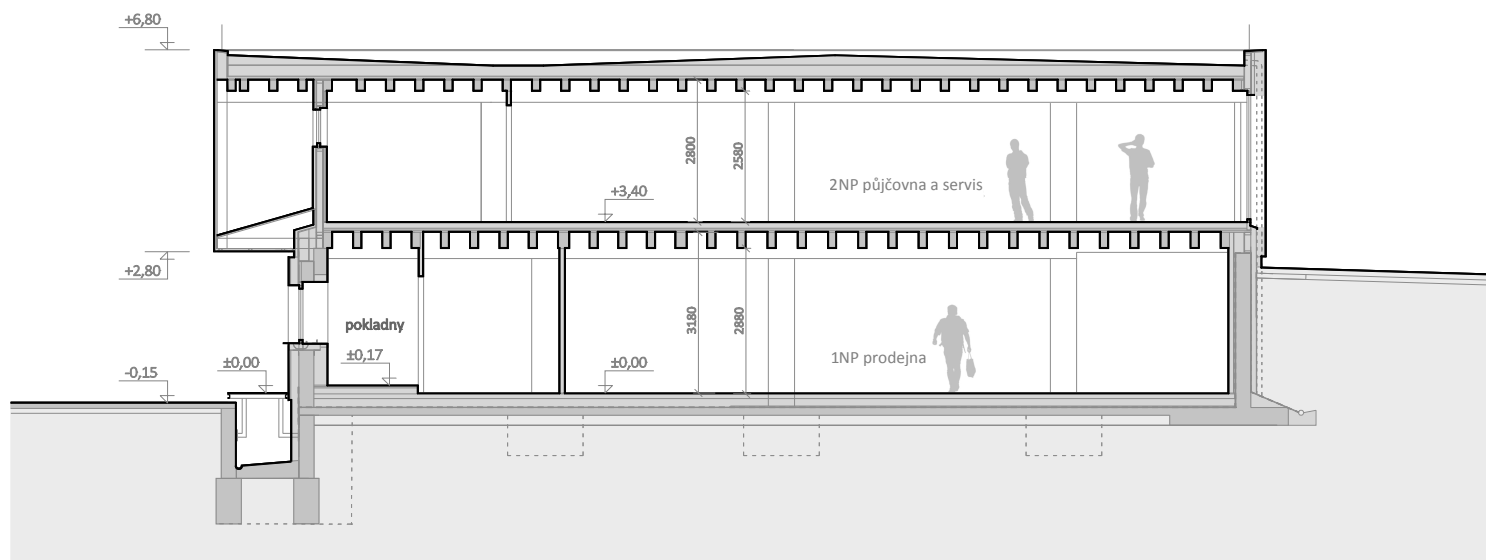
řez podélný B
