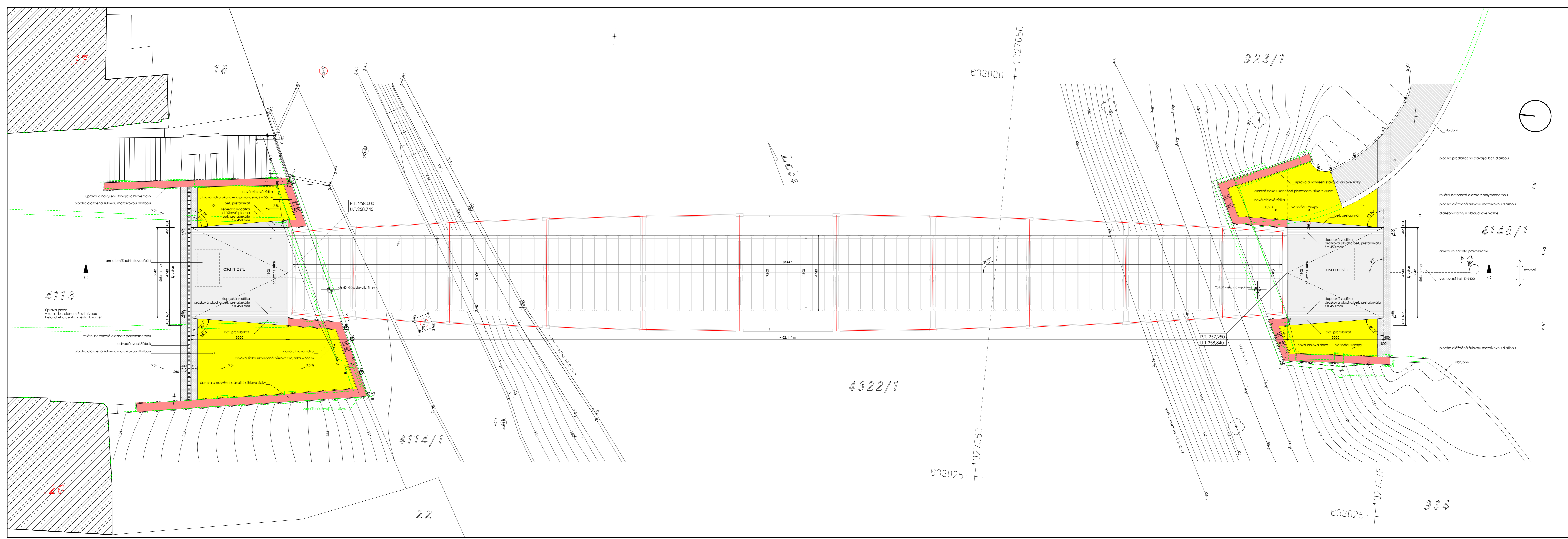
půdorys a pohled s okolím / řez terénem v ose lávky 1:100
