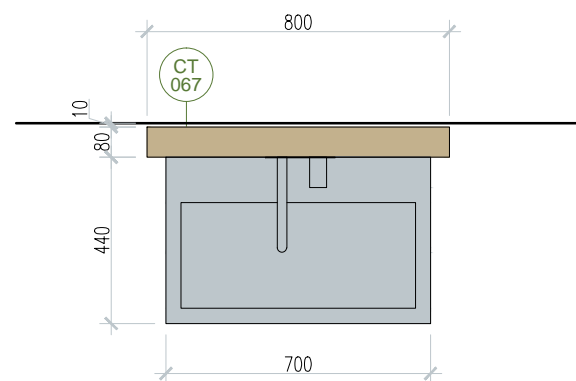
POHLED ČELNÍ
