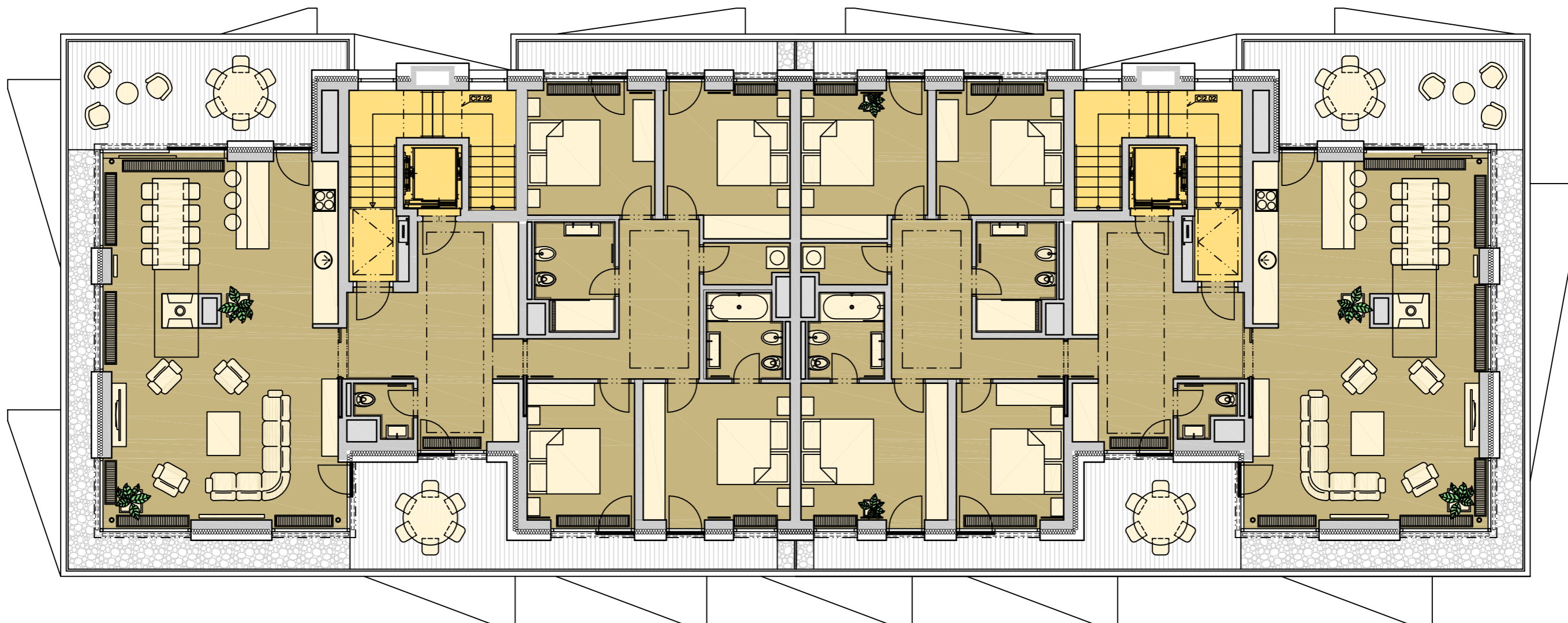
ORIENTAČNÍ SCHÉMA ETAPY I / PHASE I SCHEME
