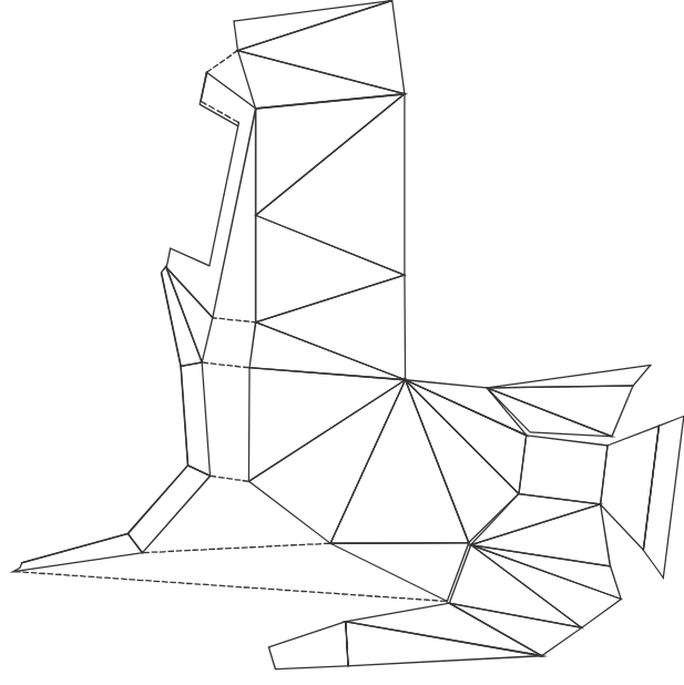
ROZVINUTÉ PLOCHY STŘECHY
