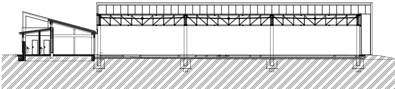
ŘEZ PRÍČNÝ
