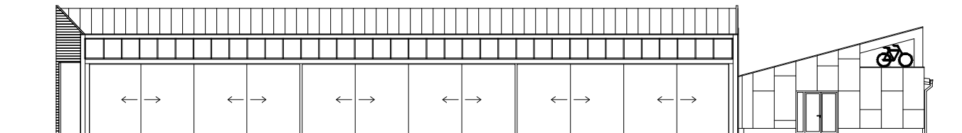
POHLED JIHOVÝCHODNÍ
