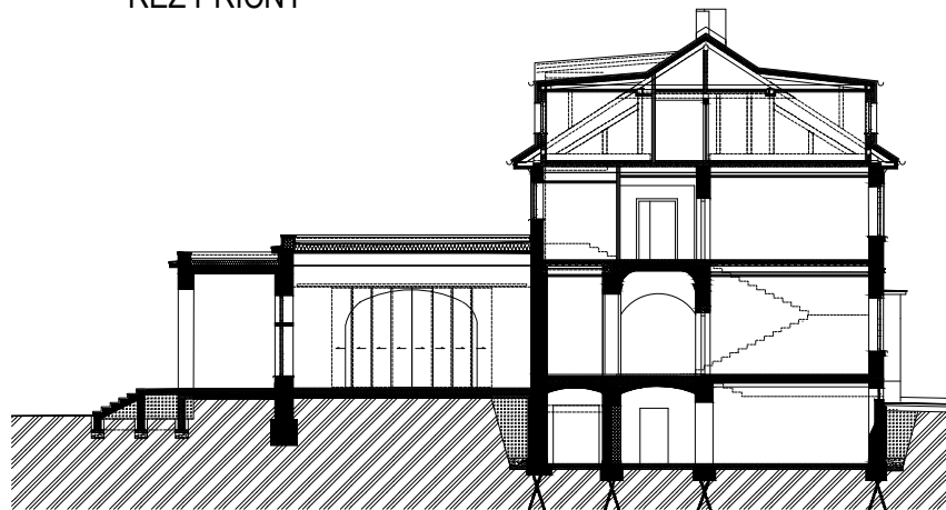
ŘEZ PŘÍČNÝ
