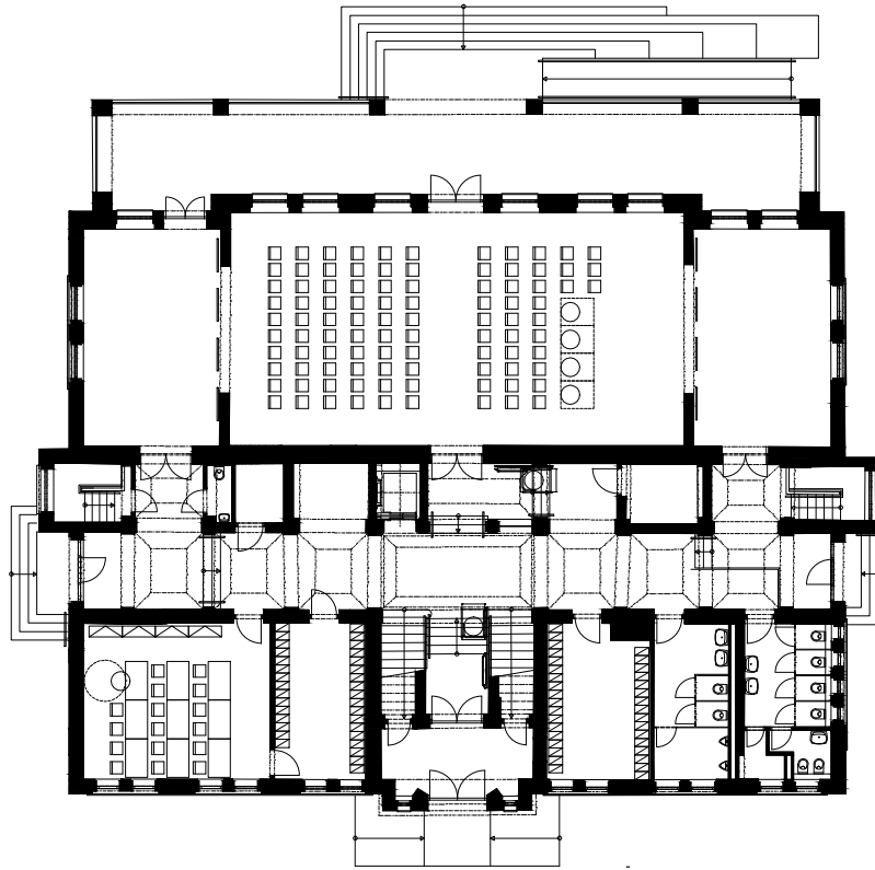
PŮDORYS 1.NP
