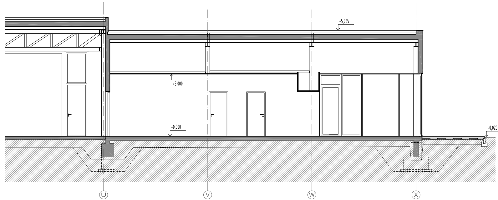
ŘEZ 1 - 1'
