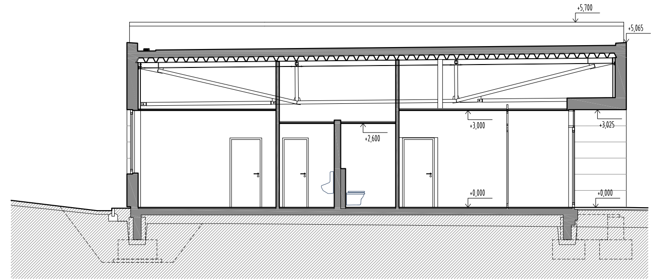
ŘEZ 3 - 3'
