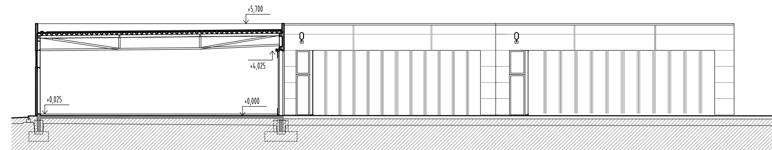
ŘEZ 2 - 2'
