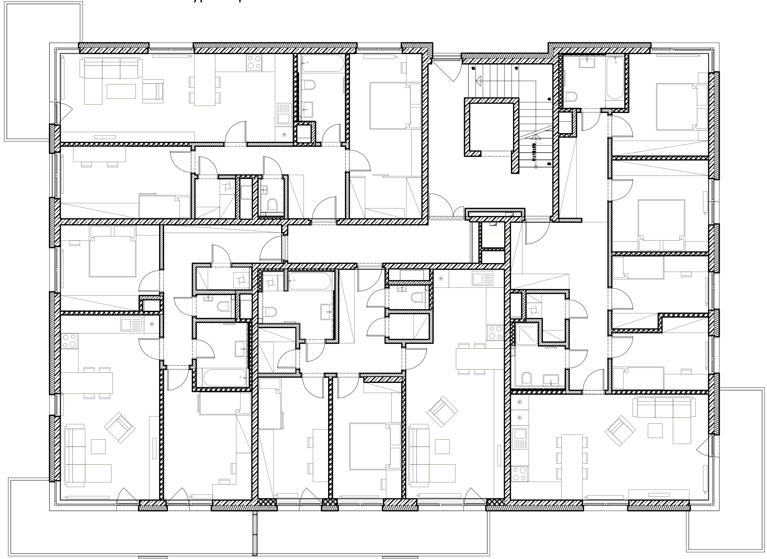
Budova C - typické podlaží
