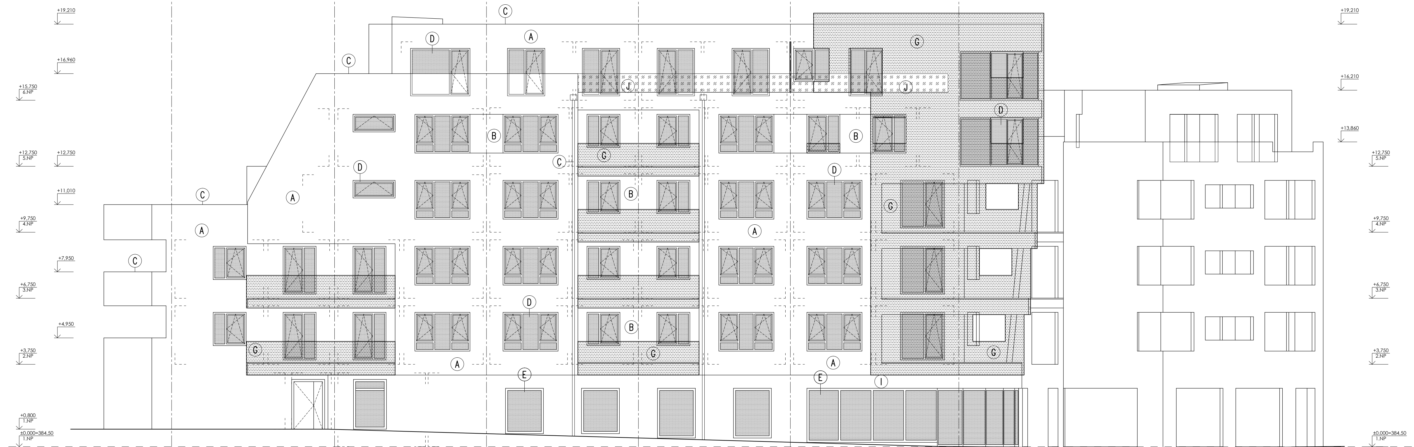
SEKCE "A" - POHLED JIŽNÍ
