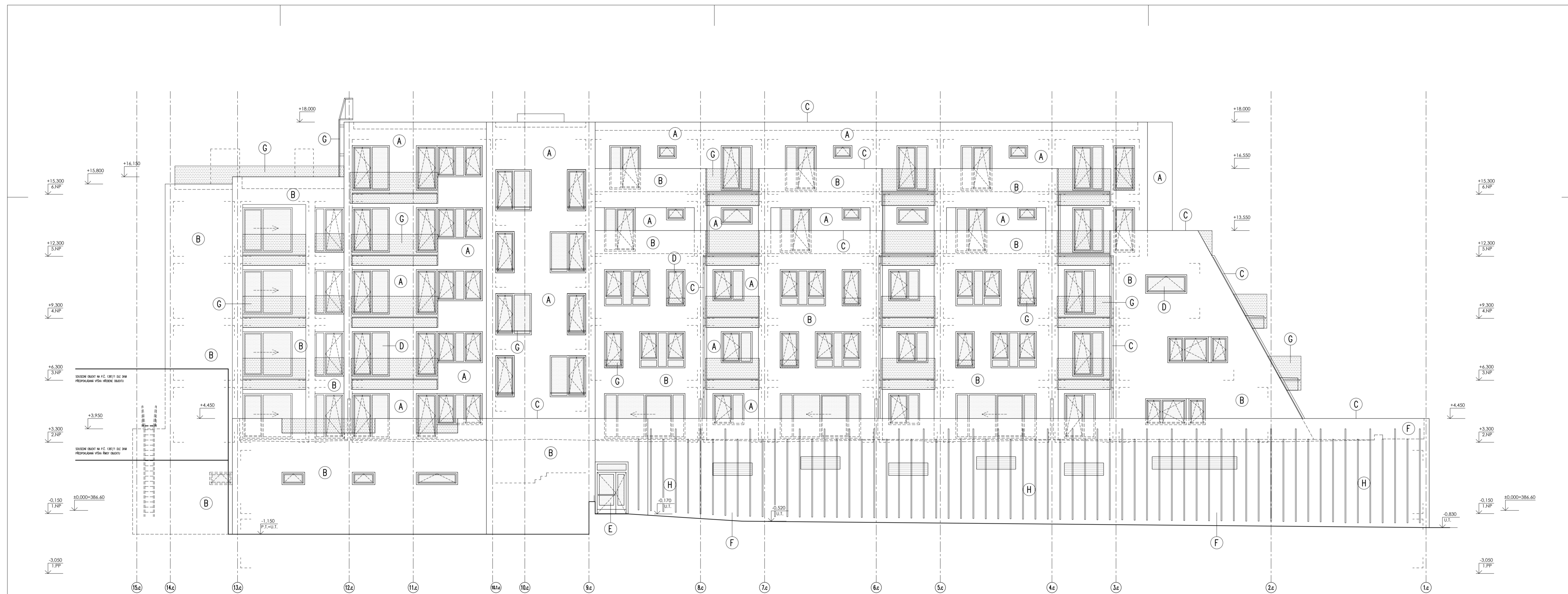
POHLED ZÁPADNÍ
