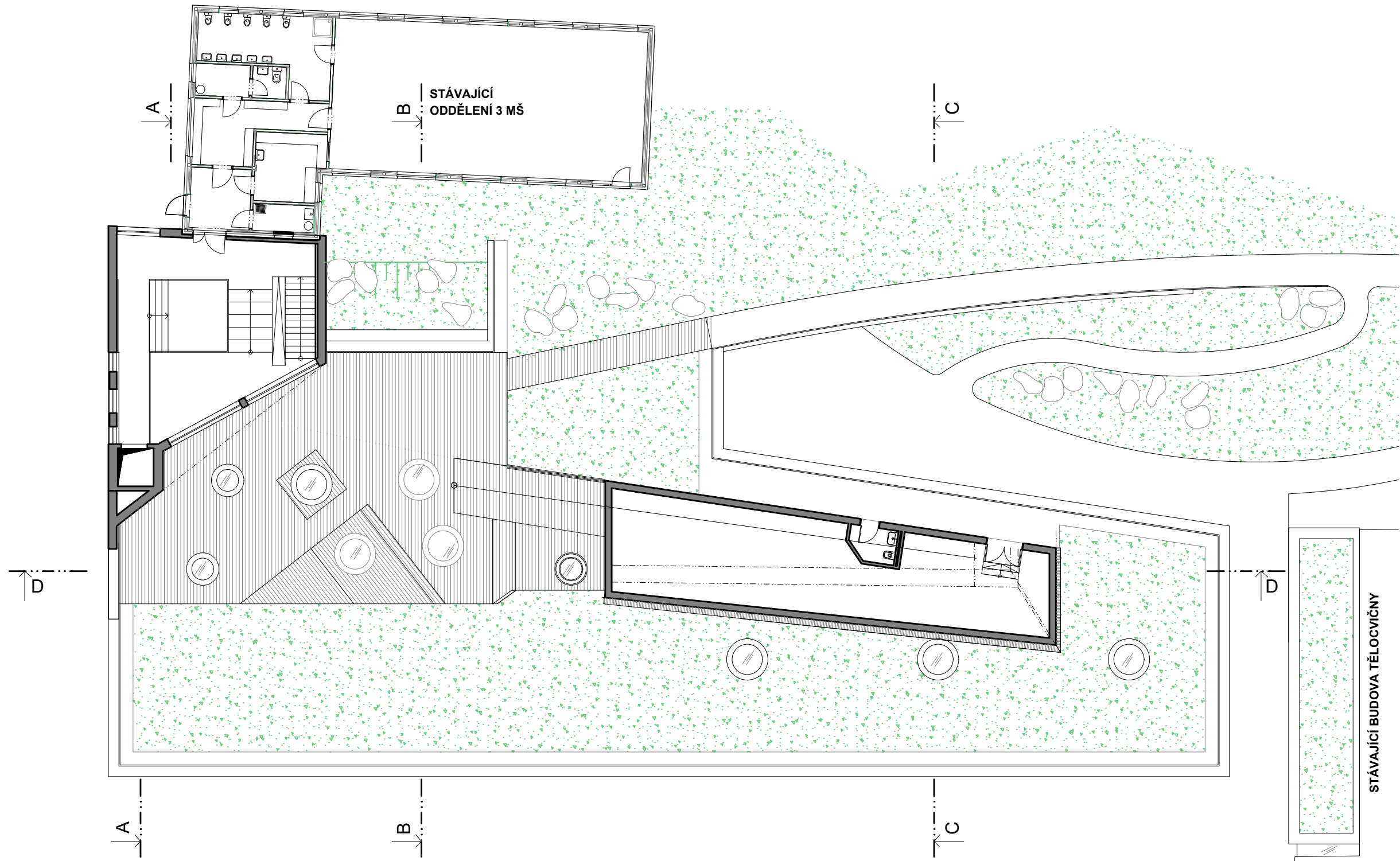
PŮDORYS 2.NP
